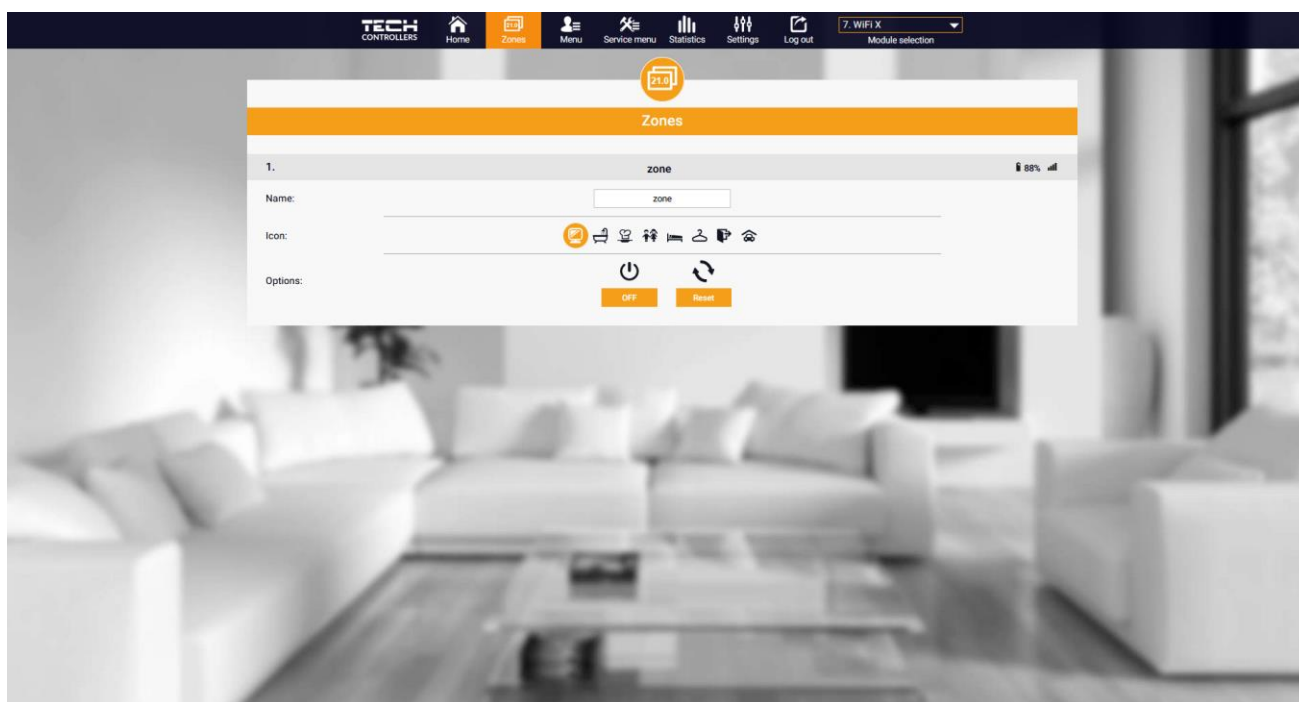
Zones tab
