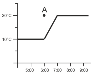
Температура в помещении - выключенная функция «ОПТИМУМ СТАРТ»
