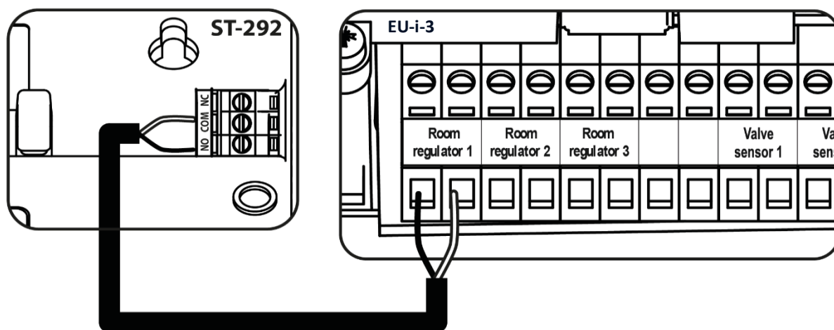
Példa kétállású szabályozó csatlakoztatására
