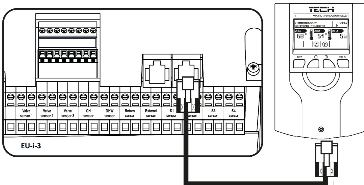
Példa: a kiegészítő szelep és az EU-i-3 fő vezérlő közötti kapcsolat
