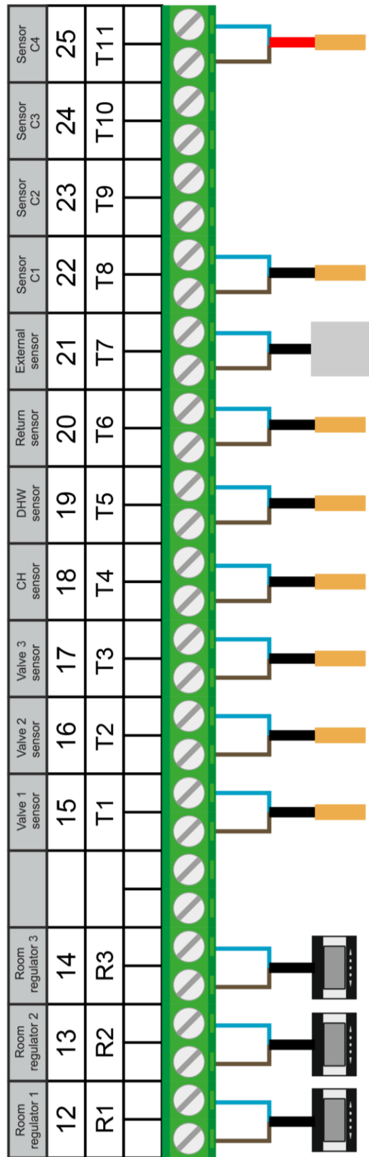
Csatlakozók, szimbólumok és felhasználási példák
