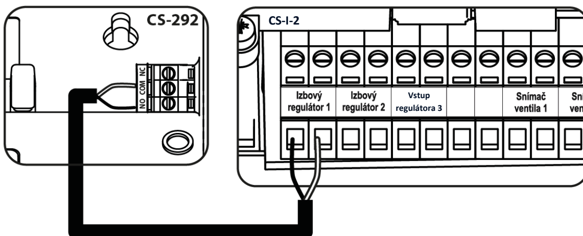
Príklad zapojenia dvojpolohového izbového regulátora (ON/OFF)
