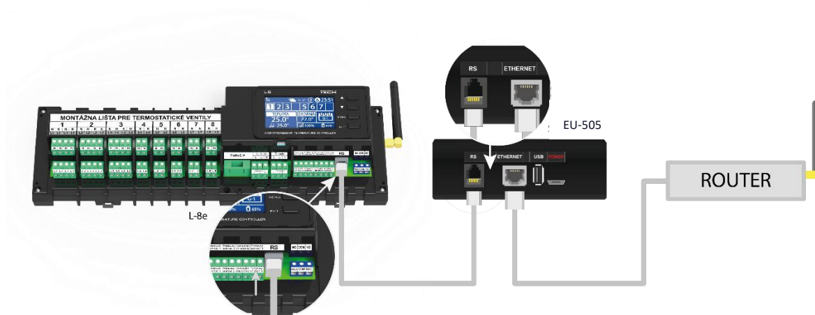
Schéma pripojenia internetového modulu EU-505.
