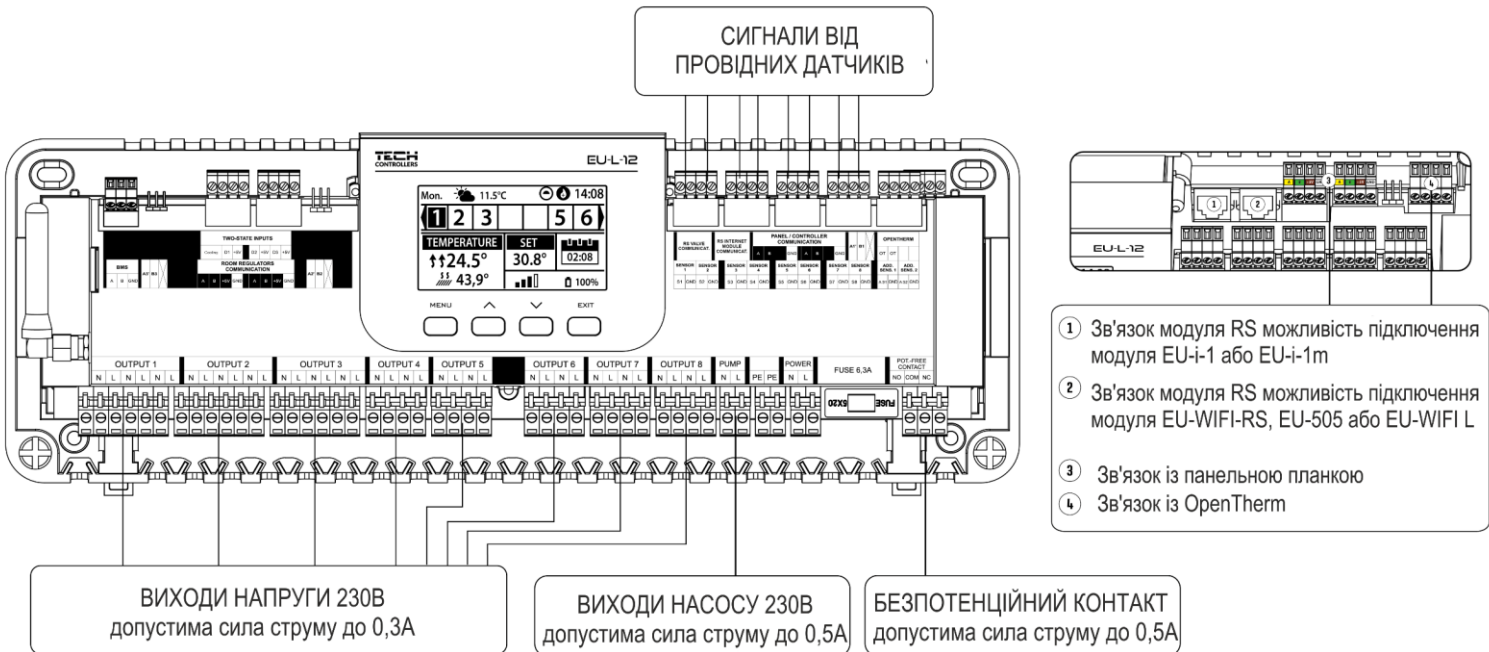
Ілюстративна схема, що показує способи підключення та зв'язку з іншим обладнанням установки:
