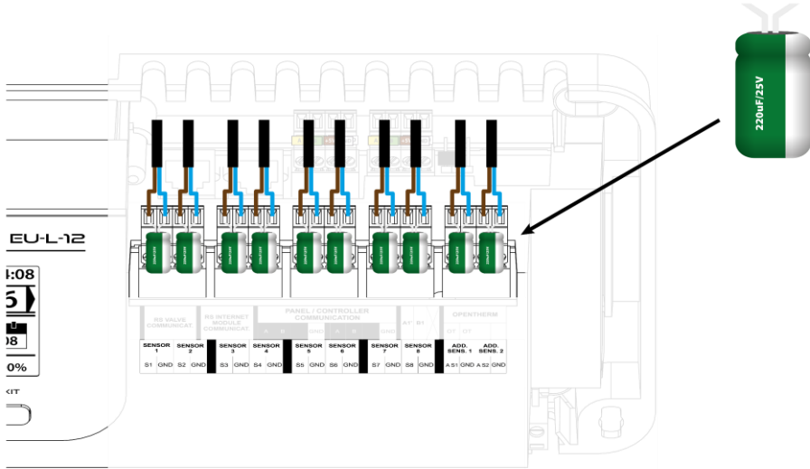
Ілюстративна схема, що показує способи підключення та зв'язку з іншим обладнанням установки:
